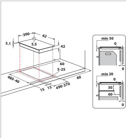
BRD 4030 B
