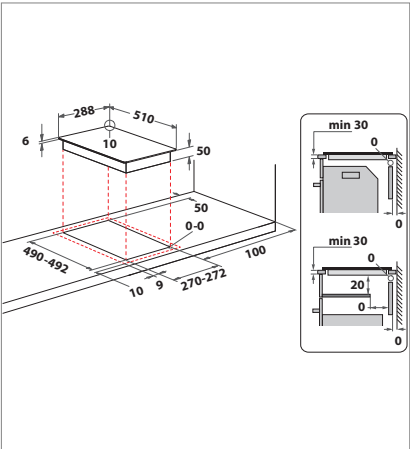
ETK 5240 IN
