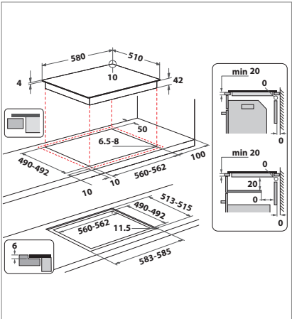
ESIS 8641 NE
