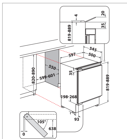
UVI 1950 LH2
