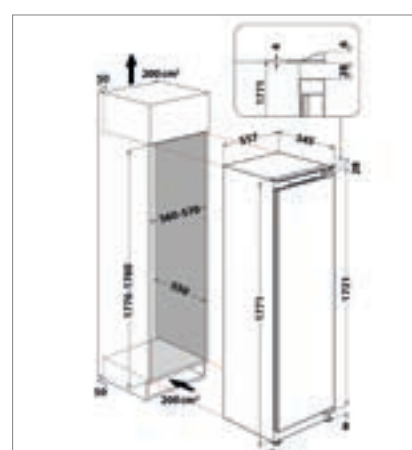
KVIS 28623
